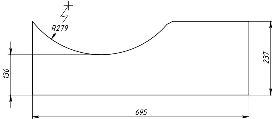
Поз.2 (Угольник)
